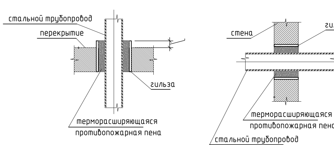
Схема устройства отверстий ВК (Схема 1)
