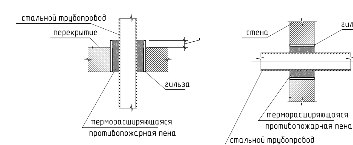
Узел проходки трубопроводов через строительные конструкции
