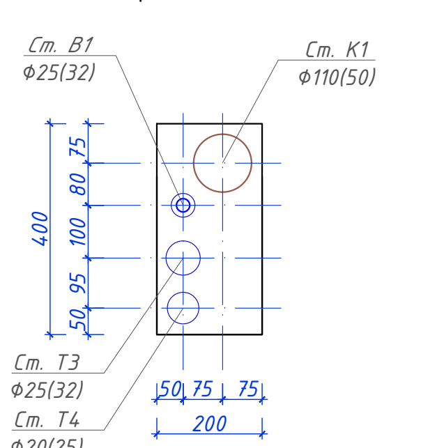
Схема устройства отверстий ВК (Схема 1)
