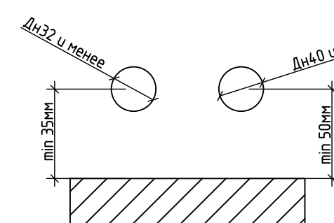
Узел проходки трубопровода через строительные конструкции
