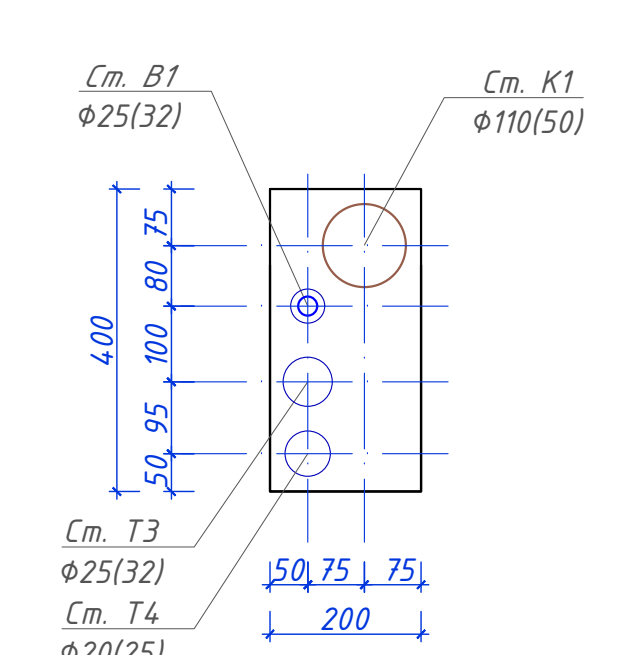
Схема устройства отверстий ВК (Схема 1)
