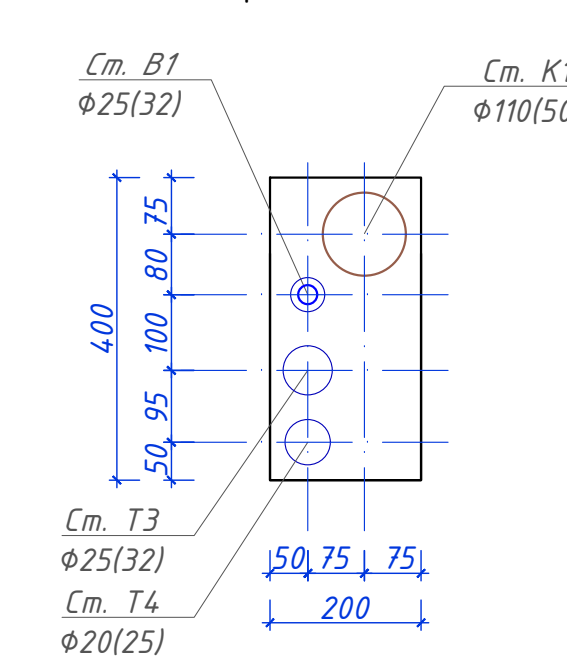
Схема устройства отверстий ВК (Схема 1)
